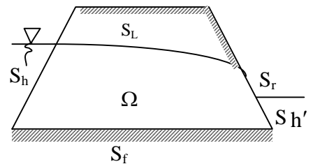
Figure .1 Conditions aux limites dans un barrage en terre homogène
