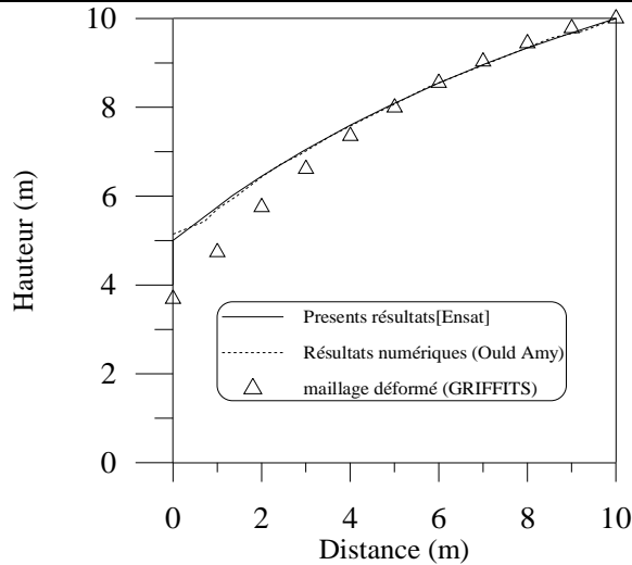
Fig.4 Ecoulement permanent dans un barrage homogène carré
