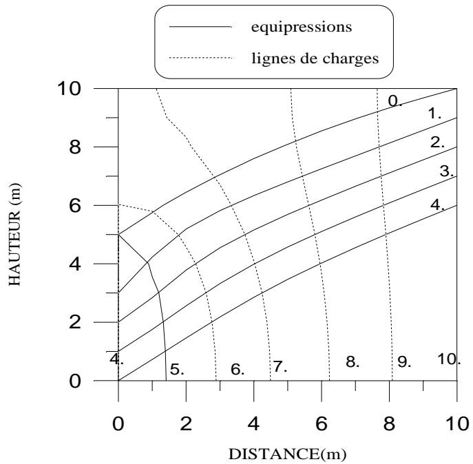
Fig .9 Lignes d'équipression et lignes de charge dans un barrage rectangulaire
