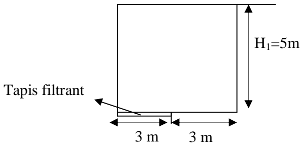
Fig.5 Ecoulement permanent dans un barrage homogène à tapis filtrant
