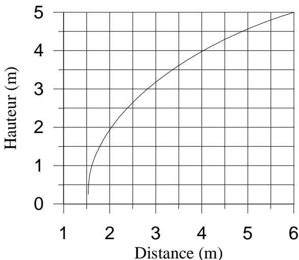
Fig.6 Ecoulement permanent dans un barrage homogène à tapis filtrant
